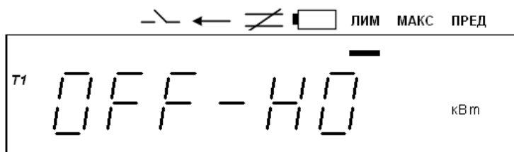
Рисунок 4.25 – Индикация превышения лимита мощности
