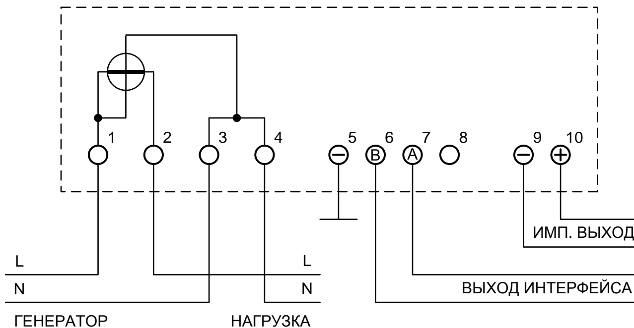
Рисунок Б.1 – Схема подключения счетчика
