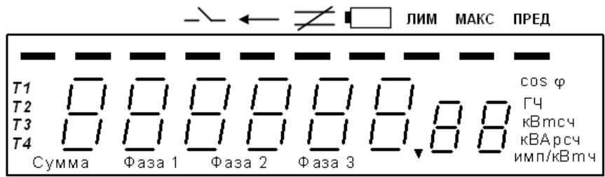
Рисунок 4.9 – Внешний вид ЖКИ
