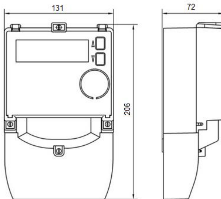
Рисунок А.1 – Габаритный чертеж счетчика
