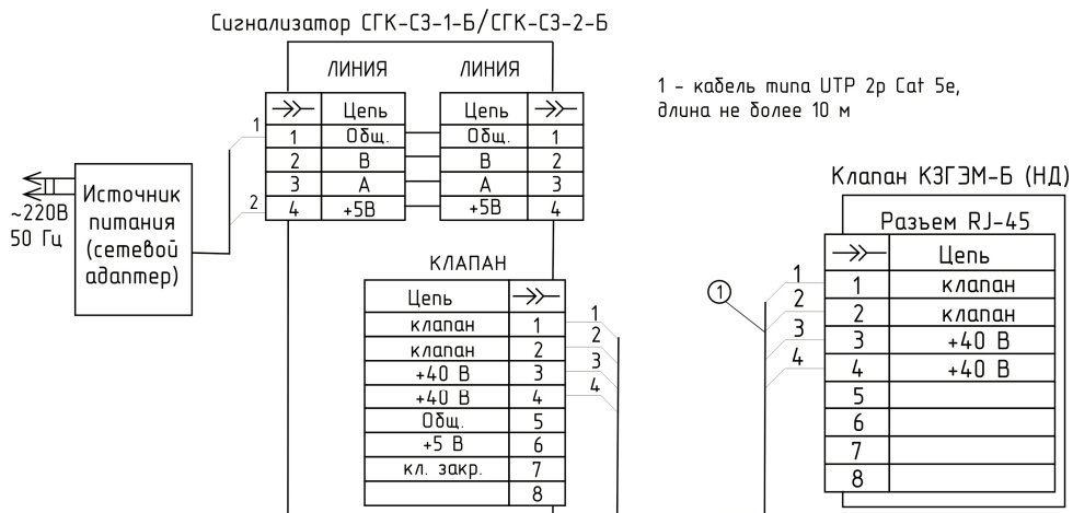
Рис. 2. Схема электрических соединений сигнализаторов SGK-S3-x-B и бытового электромагнитного клапана КЗГЭМ-Б(без узла индикации положения клапана).
