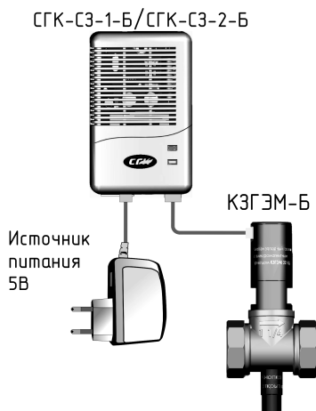
Рис. 1. Сигнализаторы SGK-S3-x-B с клапаном типа КЗГЭМ-Б.
